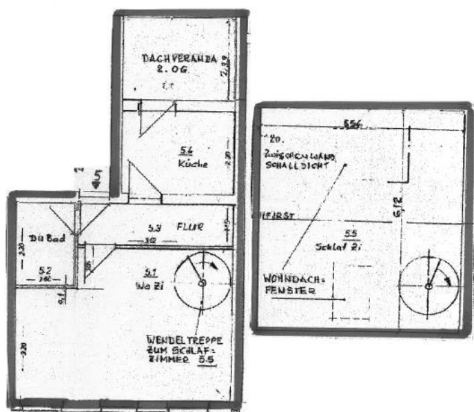
2. Obergeschoss / Mansardgeschoss
